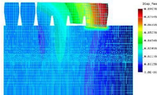
Ryc. 11. Odwzorowanie przesunięcia mostu z podparciem szklanym przy obciążeniu prostopadłym 100 N
