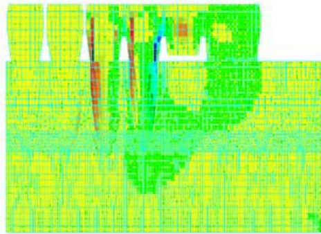
Ryc. 6. Odzworowanie prostopadłego naprężenia rozciągającego i ściskającego przy zastosowaniu podparcia szklanego
