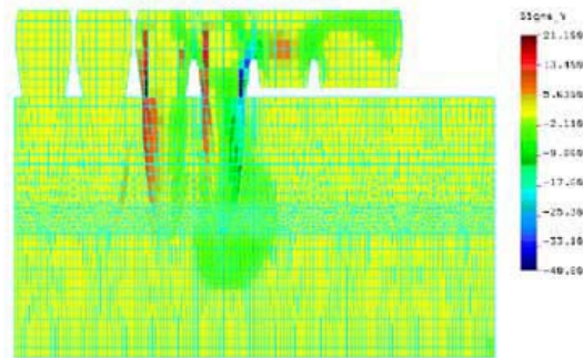
Ryc. 7. Odzworowanie prostopadłego naprężenia rozciągającego i ściskającego w moście niepodpartym
