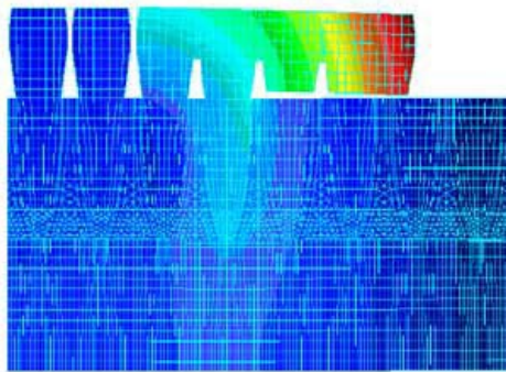
Ryc. 10. Odwzorowanie przesunięcia mostu niepodpartego przy obciążeniu prostopadłym 100 N
